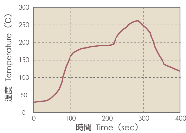
◎リフロープロファイル Reflow profile
