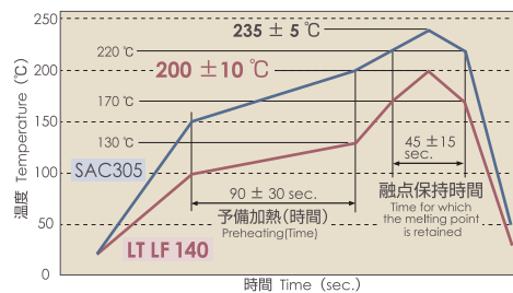
◎リフロープロファイル Comparison of reflow profile
