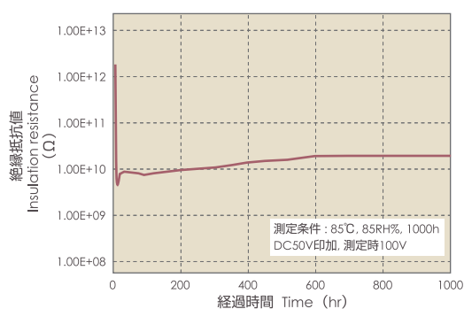
◎マイグレーション試験 Electromigration test
